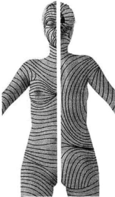
Рисунок 1. Лінії Лангера
